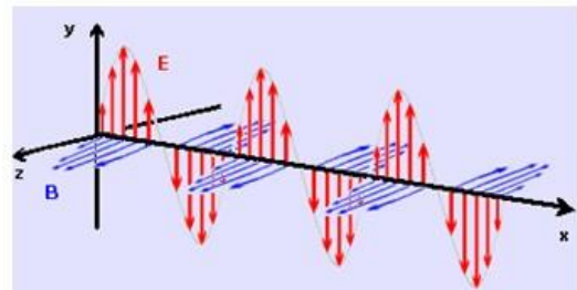
Figura 2: Representação instantânea dos vetores campos elétricos (verticais) e magnéticos (horizontais) de uma onda eletromagnética.
